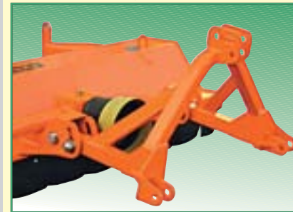
Attacco a tre punti. Three-point-hitch. Attelage à trois points. Drei-Punkt-Anbau. Conexión a tres puntas.
